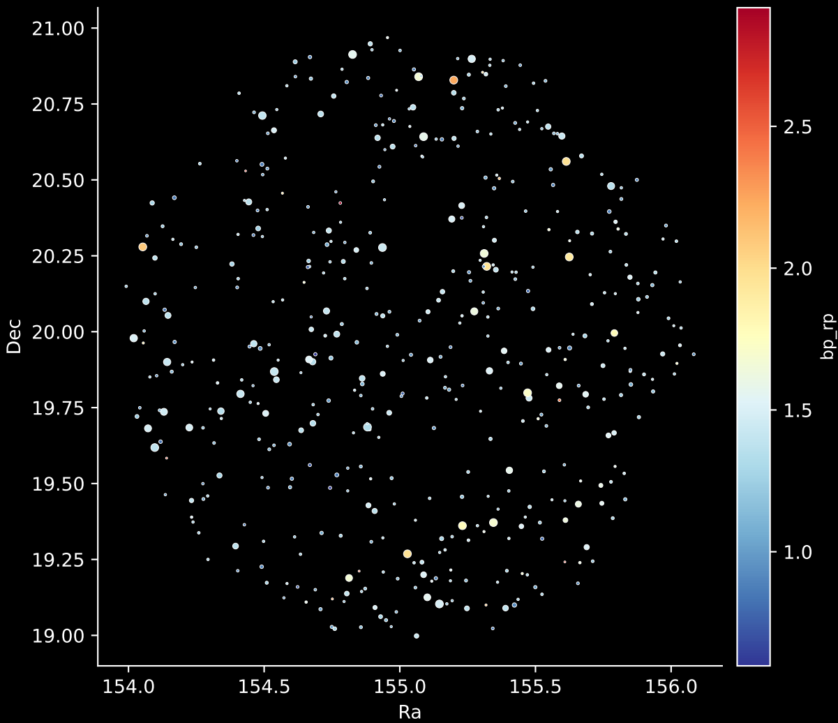
GALAH DR4 Field: [6598] Stars: 478
