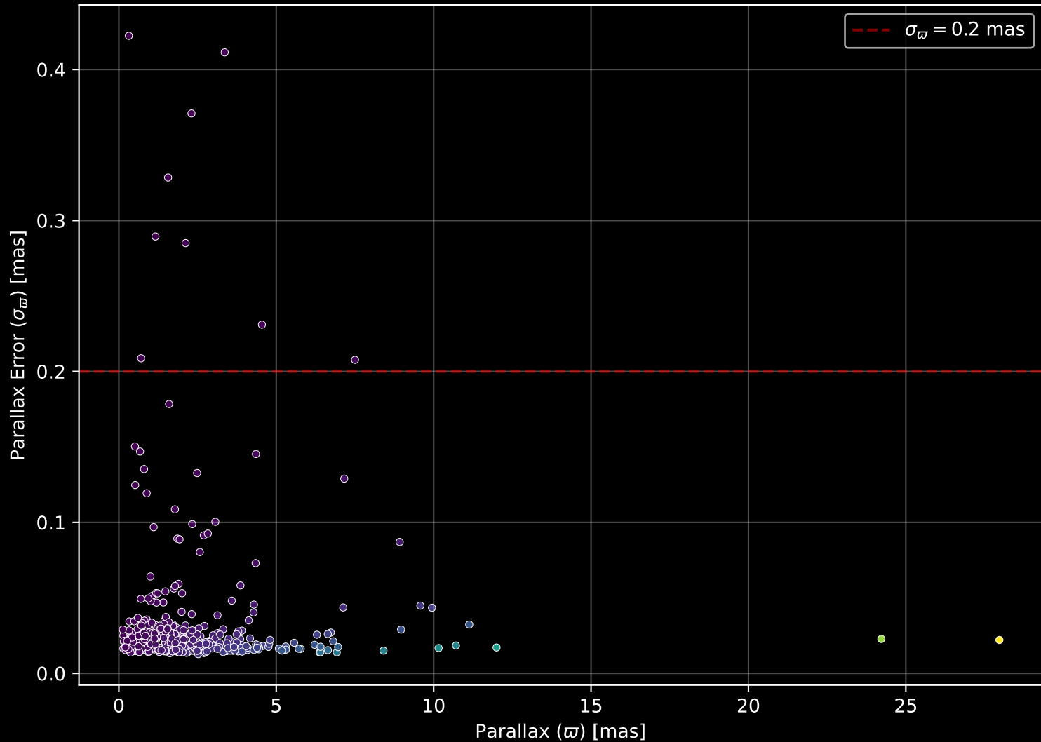
GALAH DR4 Field: [6598] Parallax Quality (n= 478)
