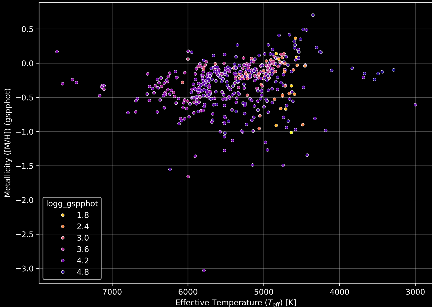
GALAH DR4 Field: [6598] Stellar Population Parameters (n= 478)
